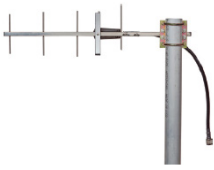
Yagi Antenna 900MHz
